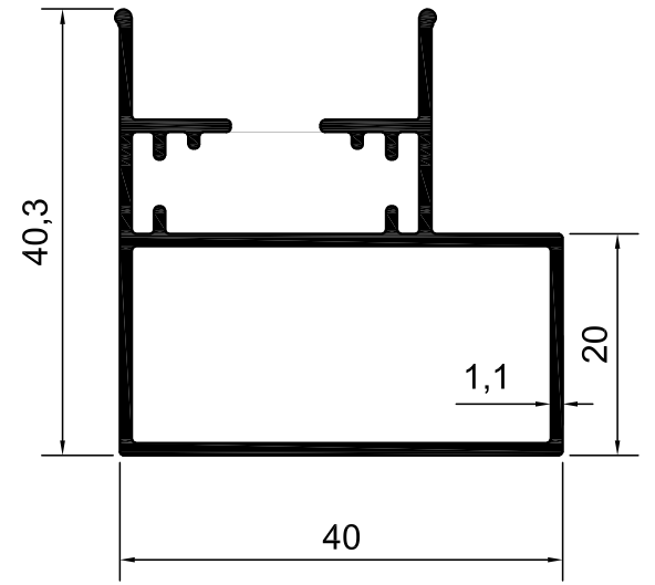
KOD-1005 TEORİK AĞIRLIK-0,553 KG/M
