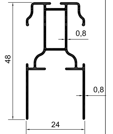
KOD-1023 TEORİK AĞIRLIK-0,360 KG/M
