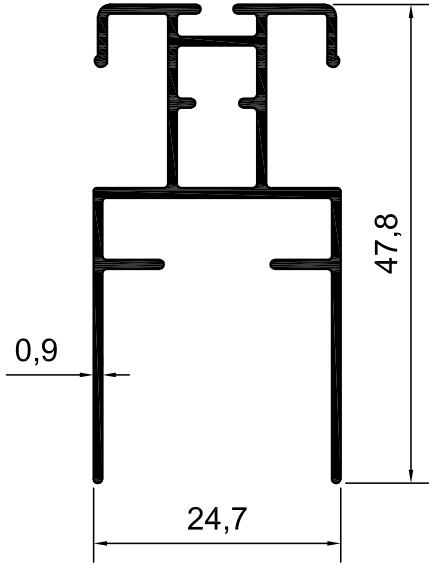
KOD-1021 TEORİK AĞIRLIK-0,425 KG/M
