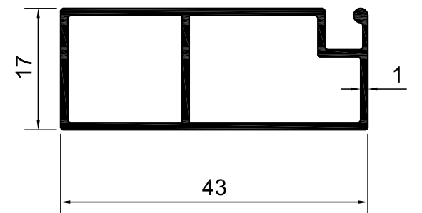
KOD-1035 TEORİK AĞIRLIK-0,371 KG/M
