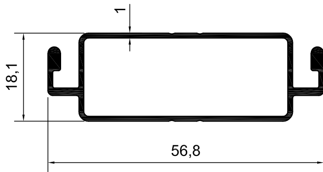
KOD-1015 TEORİK AĞIRLIK-0,453 KG/M
