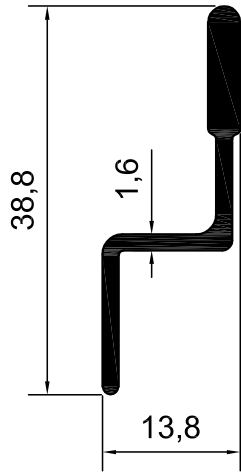
KOD-1012 TEORİK AĞIRLIK-0,268 KG/M
