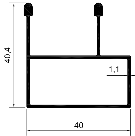
KOD-1040 TEORİK AĞIRLIK-0,590 KG/M
