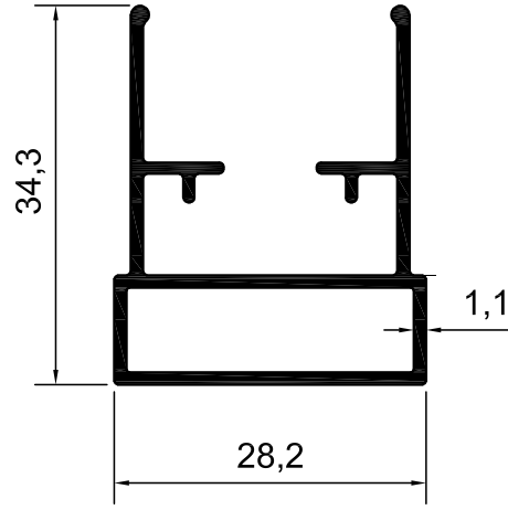
KOD-1010 TEORİK AĞIRLIK-0,415 KG/M
