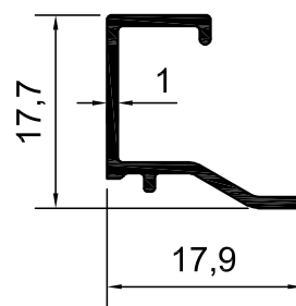
KOD-1019 TEORİK AĞIRLIK-0,121 KG/M
