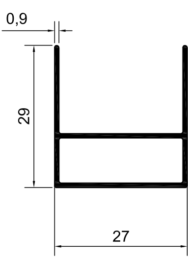
KOD-1024 TEORİK AĞIRLIK-0,264 KG/M
