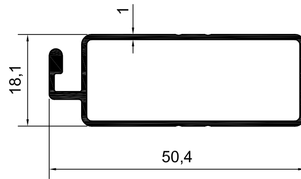
KOD-1014 TEORİK AĞIRLIK-0,385 KG/M
