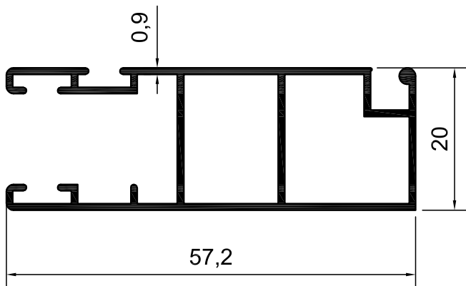
KOD-1011 TEORİK AĞIRLIK-0,493 KG/M
