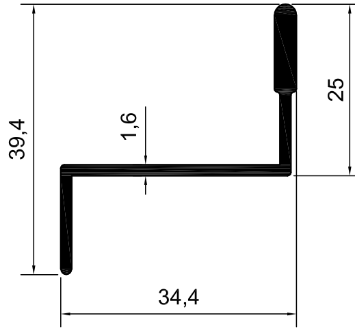
KOD-1013 TEORİK AĞIRLIK-0,361 KG/M
