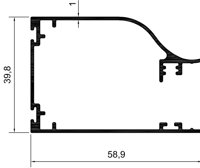
KOD-1001 TEORİK AĞIRLIK-0,616 KG/M
