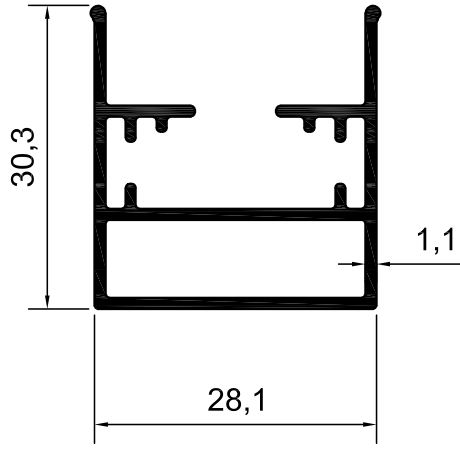
KOD-1009 TEORİK AĞIRLIK-0,423 KG/M
