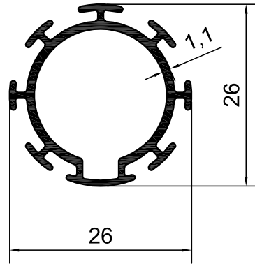
KOD-1004 TEORİK AĞIRLIK-0,304 KG/M
