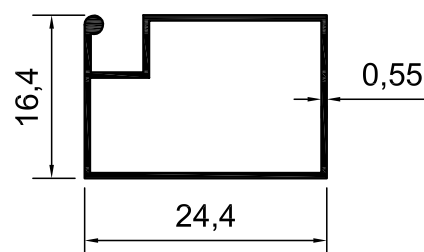
KOD-1017/B TEORİK AĞIRLIK-0,135KG/M
