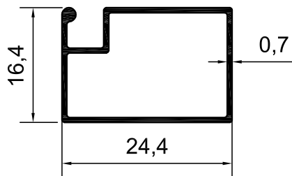
KOD-1017/A TEORİK AĞIRLIK-0,165 KG/M
