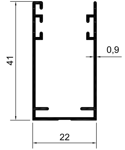
KOD-1003 TEORİK AĞIRLIK-0,318 KG/M
