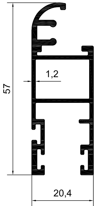
KOD-1032 TEORİK AĞIRLIK-0,688 KG/M
