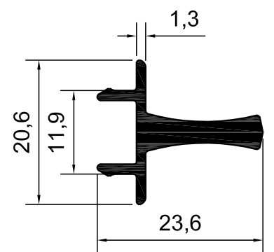
KOD-1038 TEORİK AĞIRLIK-0,280 KG/M
