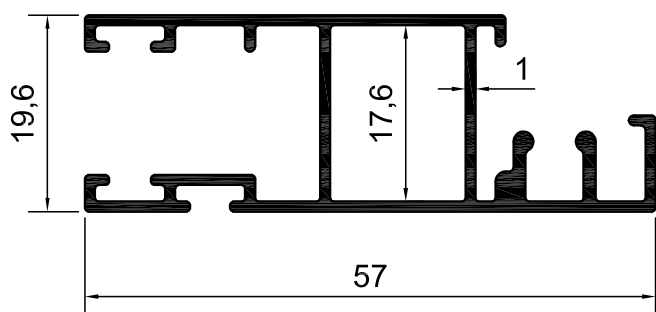
KOD-1018 TEORİK AĞIRLIK-0,523 KG/M
