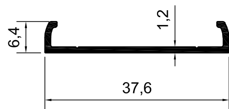
KOD-1045 TEORİK AĞIRLIK-0,161 KG/M
