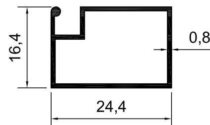
KOD-1017/C TEORİK AĞIRLIK-0,190 KG/M
