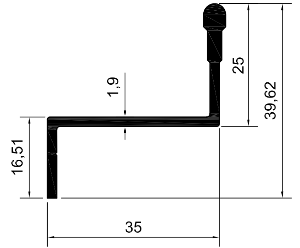
KOD-1034 TEORİK AĞIRLIK-0,422 KG/M
