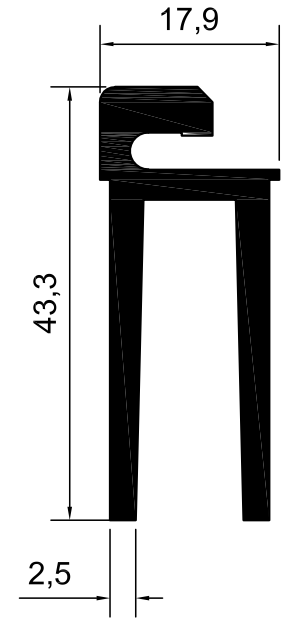
KOD-1037 TEORİK AĞIRLIK-0,817 KG/M
