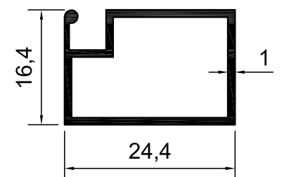
KOD-1017/D TEORİK AĞIRLIK-0,216 KG/M
