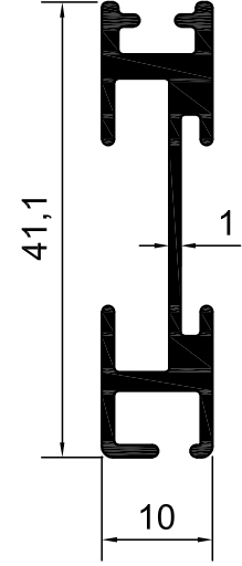
KOD-1002 TEORİK AĞIRLIK-0,377 KG/M
