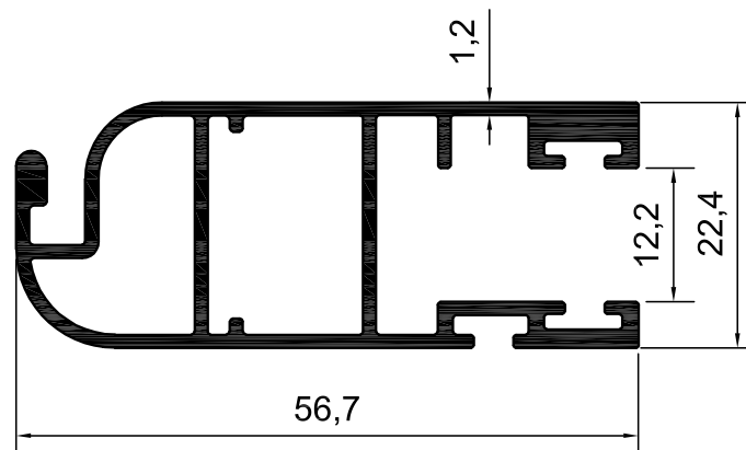
KOD-1039 TEORİK AĞIRLIK-0,771 KG/M
